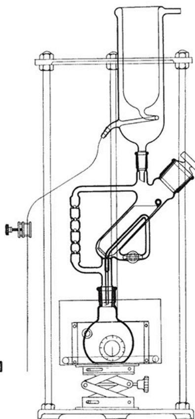
溶媒香油抽出装置
