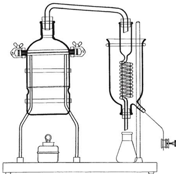
香水水蒸気蒸溜装置
